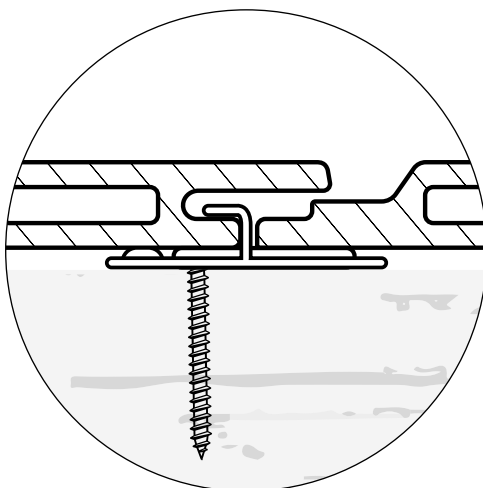
Ontzichtbare montage met hulp van RVS clip
